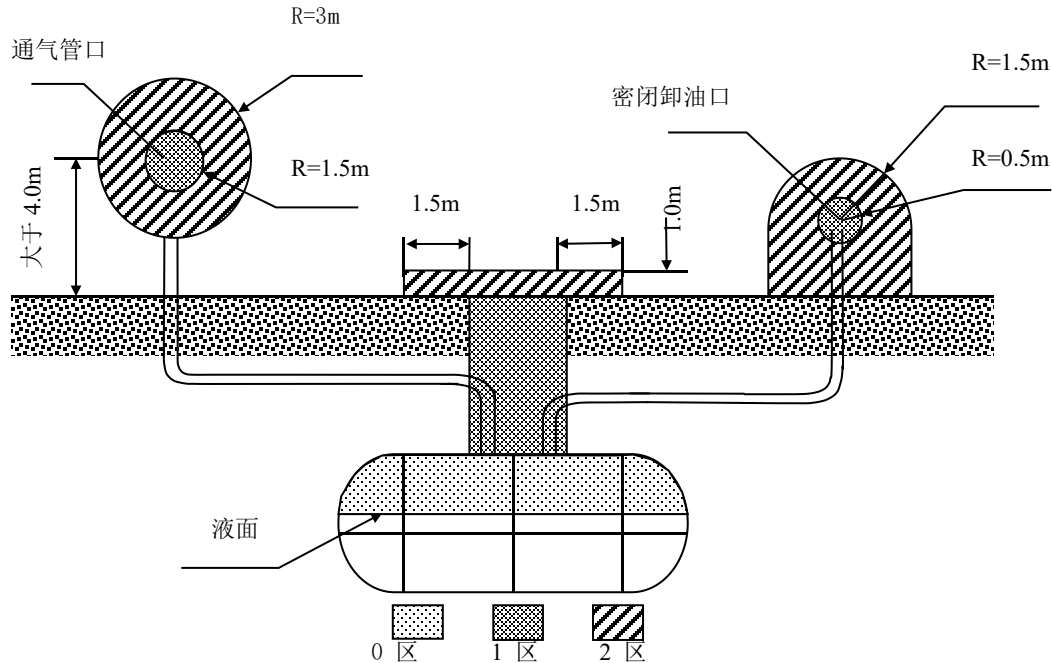
地下卧式油罐危险区域分布见下图 3：
