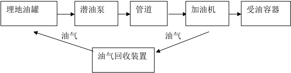
图 2.6-2 汽油加油工艺流程图
