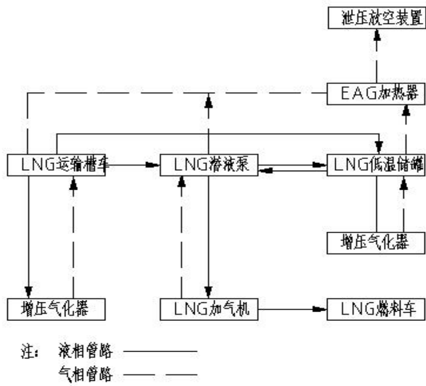
图2.7-1 LNG加气流程框图
