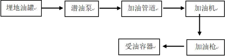
图 2.6-4 柴油加油工艺框图
