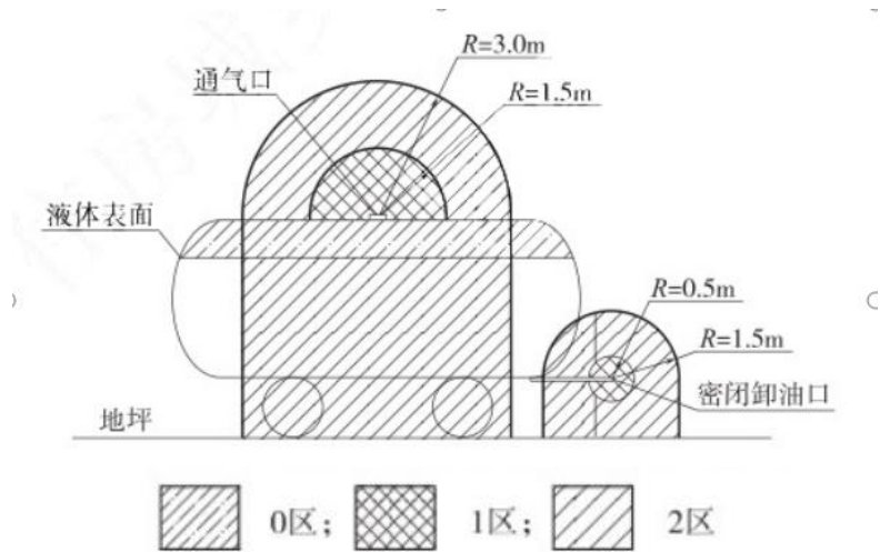
图 3.6-2 汽油储油罐车爆炸危险区域划分
